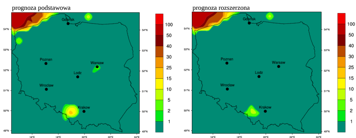
Rysunek 17. Liczba godzin z przekroczeniami progu informowania społeczeństwa 180 \mu\text{g}/\text{m}^3 dla dwóch scenariuszy redukcji emisji dla roku 2020 99
